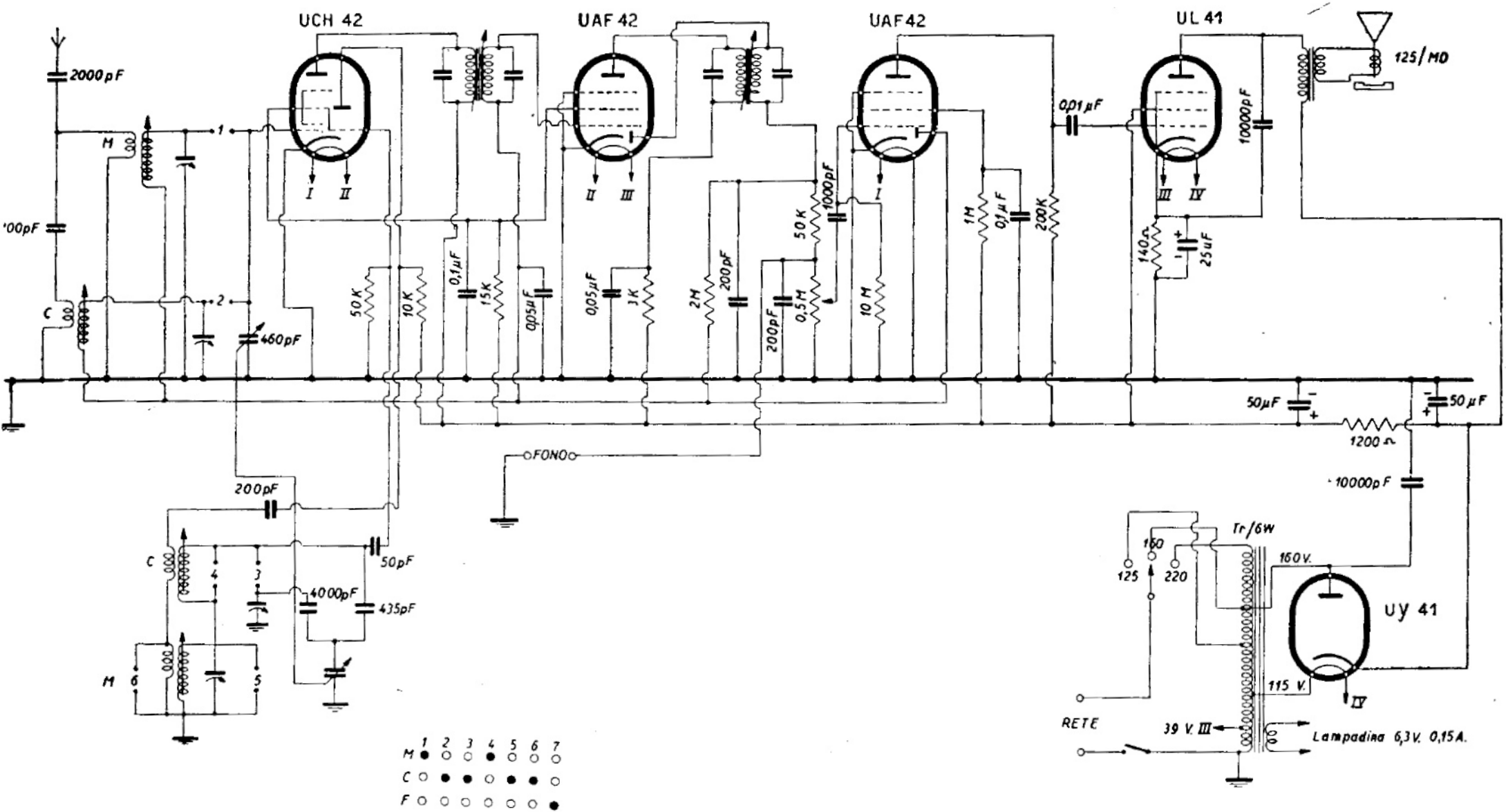
PEBA RADIO (Pertusati) - Mod. U/52 B. Gamme d'onda in metri: M 190-380 e C 16-53. Media frequenza 467 kc/s. Potenza di uscita 1 watt. Consumo 12,5 watt.
